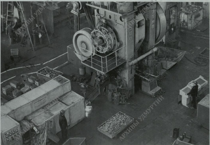
Линия горячей штамповки в кузнечном цехе Ижевского металлургического завода. 1978 г.
