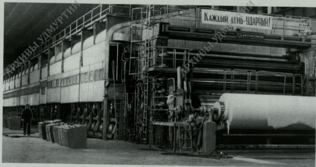
Бумагоделательная машина, изготовленная на «Ижтяжбуммаше». 1978 г.
